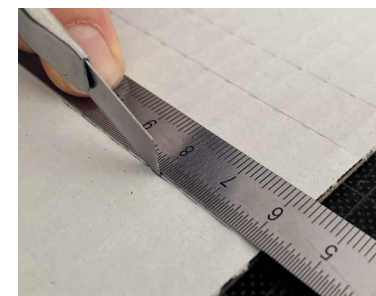
Papierkaschierung und Welle entgegen der Lafrichtung einritzen
